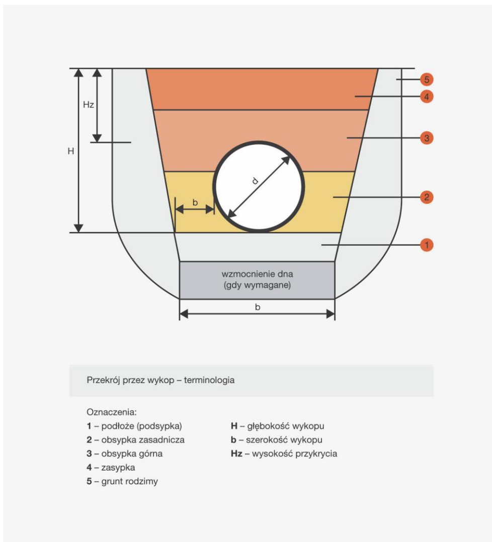
Rys. 1 Przekrój poprzeczny - terminologia
