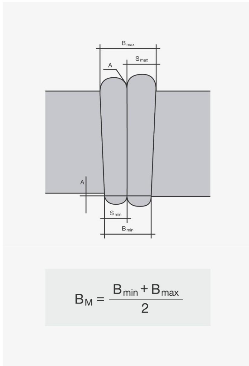
Rysunek 5. Schemat badania poprawnego połączenia
