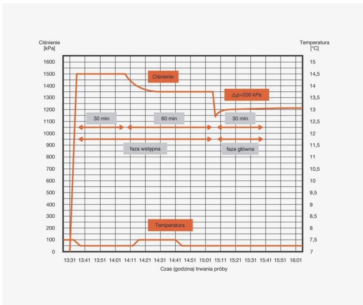
Rysunek nr 3. Przykładowy schemat próby ciśnieniowej
