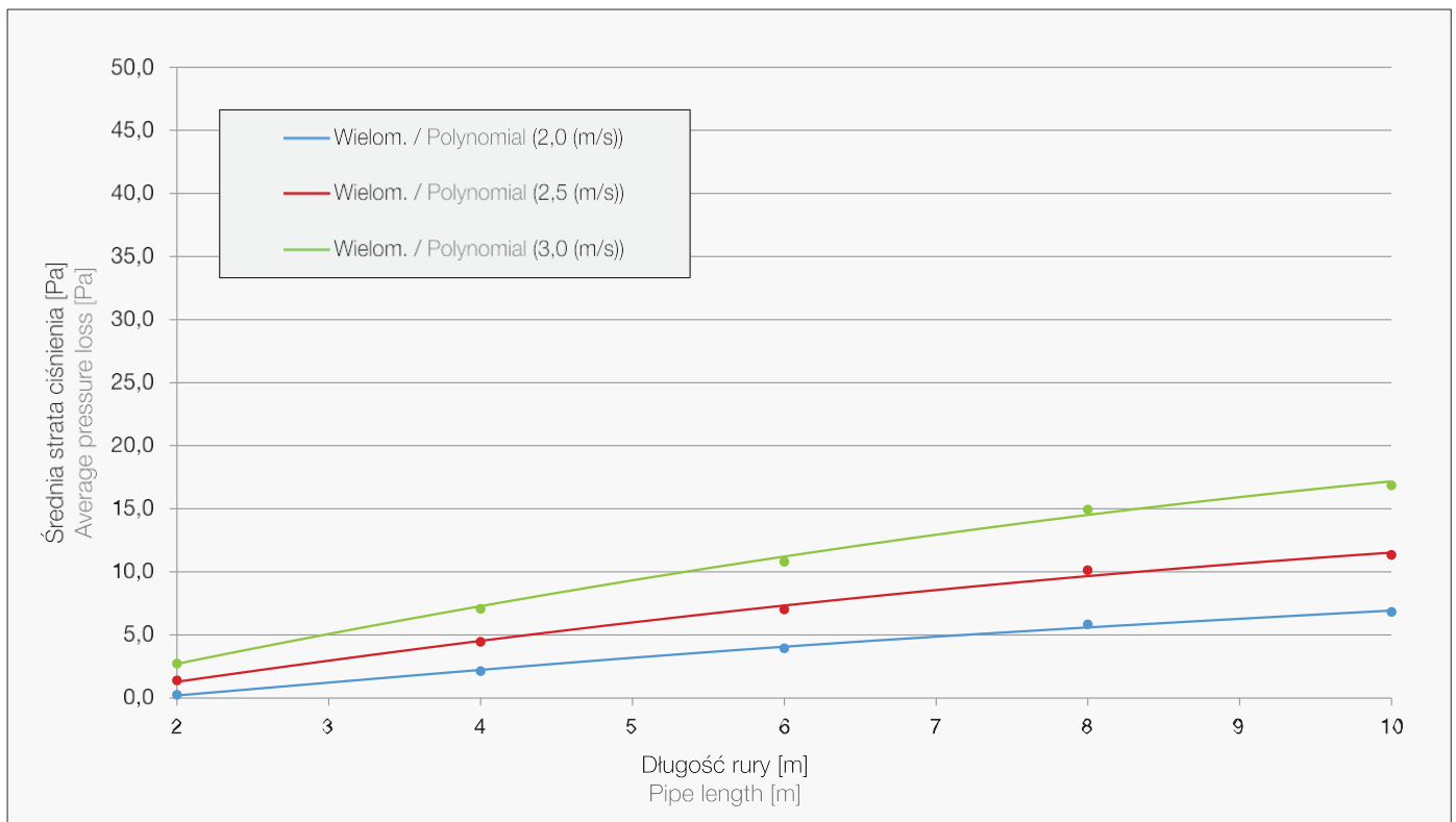
Rura wentylacyjna DN 110 / Ventilation pipe DN 110
