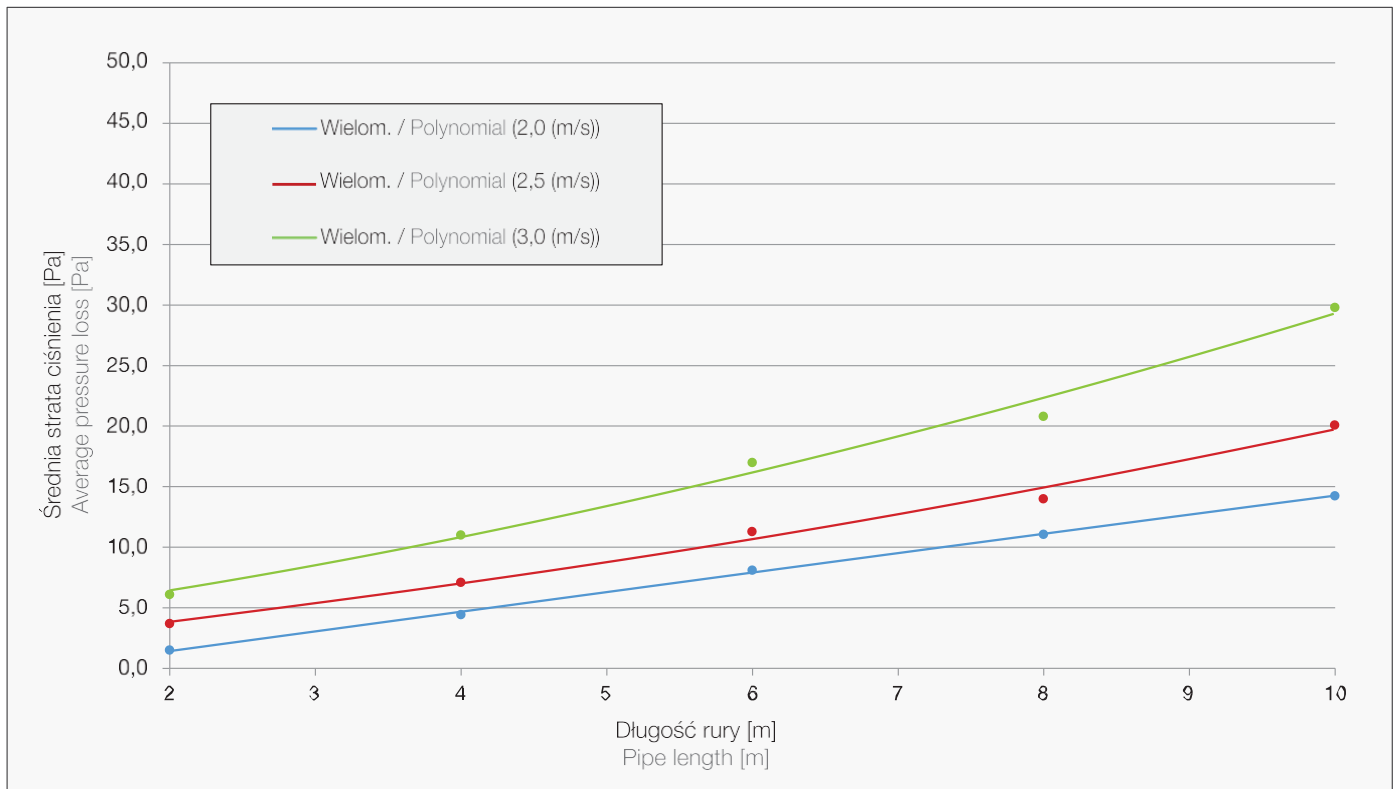
Rura wentylacyjna DN 90 / Ventilation pipe DN 90
