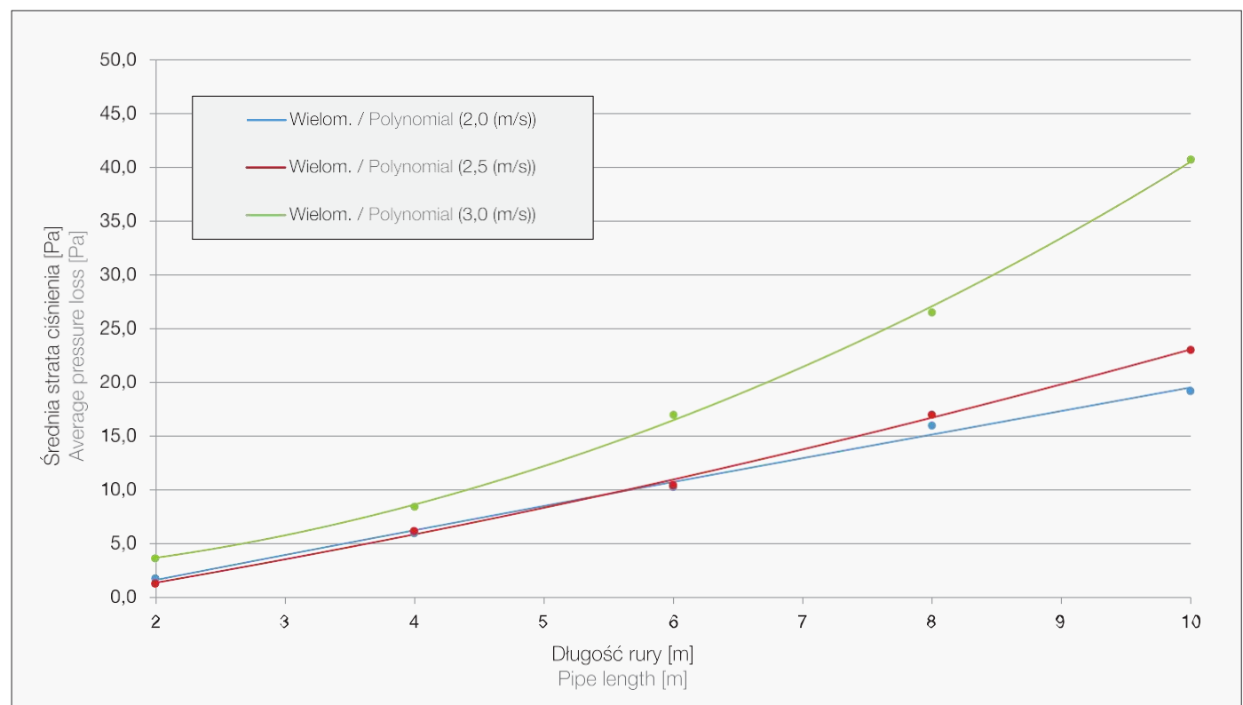
Rura wentylacyjna DN 50 / Ventilation pipe DN 50
